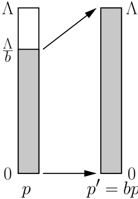
Fig. 34.6 Rescaling the momentum.
